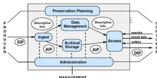
OAIS Referenz-Modell CCSDS 650.0-B-1, 2002
